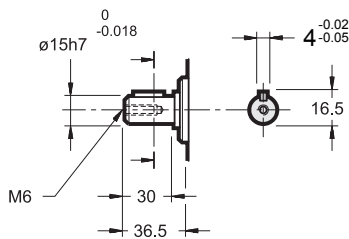
цилиндрический вал со шпонкой (идентификационный код 5)
