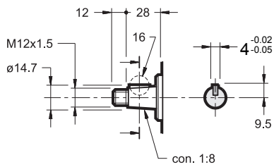
Конический вал со шпонкой (стандартный, идентификационный код 7)
