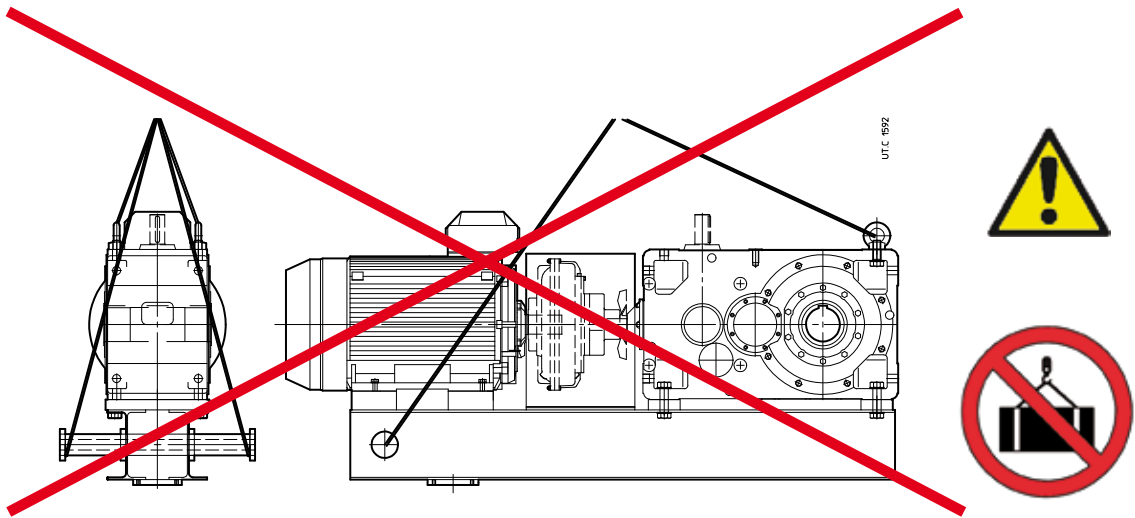
Fig. 1b - Sollevamento errato Fig. 1b - Wrong way of lifting
