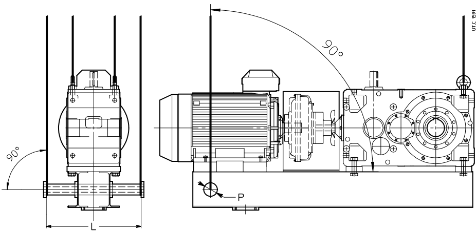
Fig. 1a - Sollevamento corretto Fig. 1a - Right way of lifting
