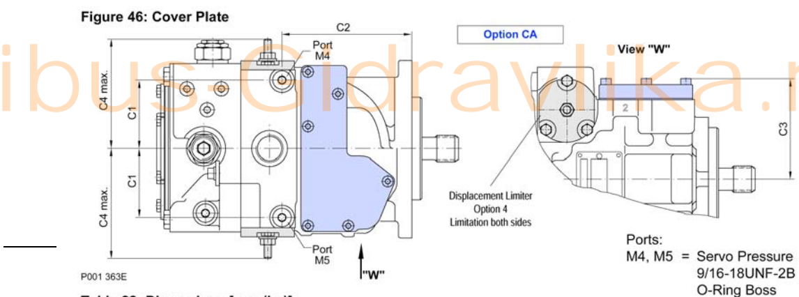
Рис. 46: Крышка
