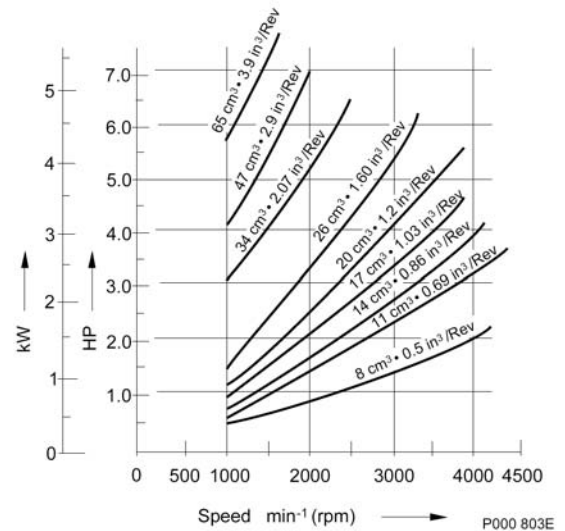
Рис. 15: Потребная мощность подкачивающего насоса
