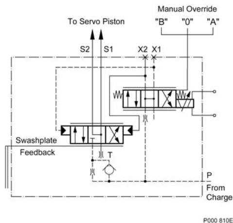
Рис. 26: Поперечное сечение клапана электрической системы управления ходом
