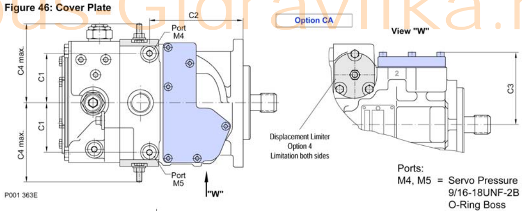
Рис. 46: Крышка
