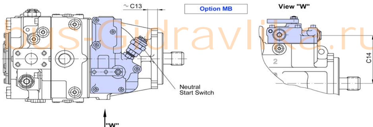
Рис.50: Система ручного управления ходом (MDC) с переключателем нейтрального положения
