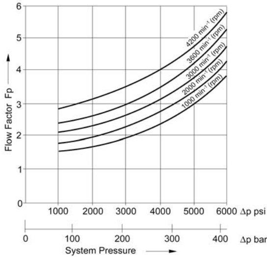
Рис. 12: Потребный расход - насос
