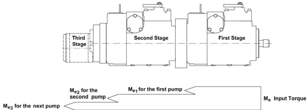
Рис. 16: Крутящие моменты для тандемного варианта крепления
